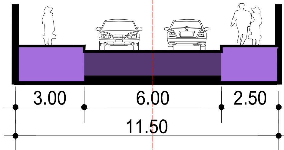
Profil Str. Gh. Lazar, scara 1/100
