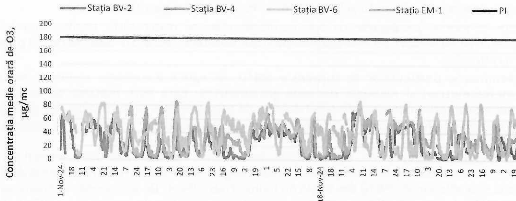
Figura 6. Evoluția concentrațiilor medii orare de O 3 în luna noiembrie 2024
