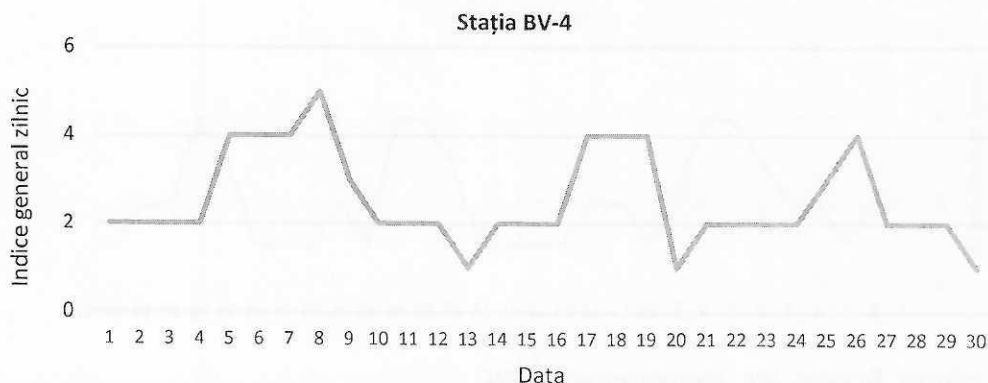
Figura 15. Evoluția indicelui general de calitate a aerului din stația BV-4
