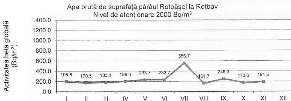
Figura 24. Activitatea beta globală la 5 zile pentru apa de suprafață-Pârâul Rotbășel
