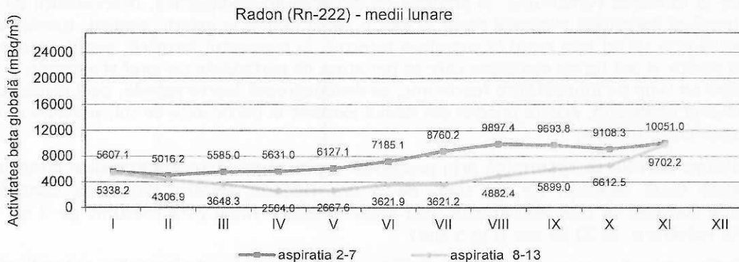
Figura 20. Activitatea calculată a Radonului
