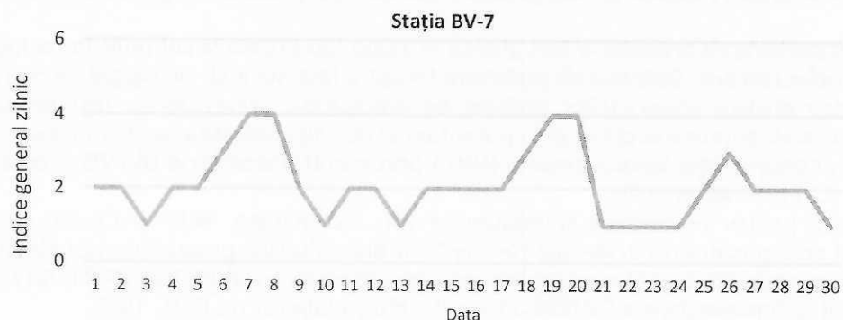
Figura 18. Evoluția indicelui general de calitate a aerului din stația BV-7
