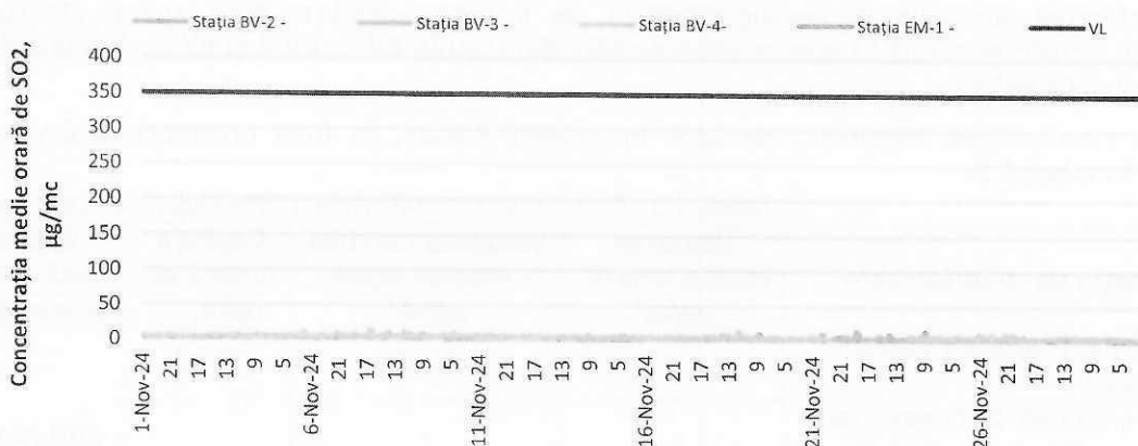
Figura 2. Evoluția mediilor orare de SO 2 în luna noiembrie 2024
