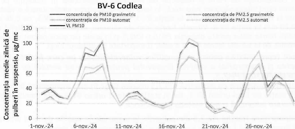
Figura 11. Evoluția concentrațiilor medii zilnice de PM10 gravimetric și automat și PM2,5 gravimetric și automat în stația de fond urban BV-6 în luna noiembrie 2024
