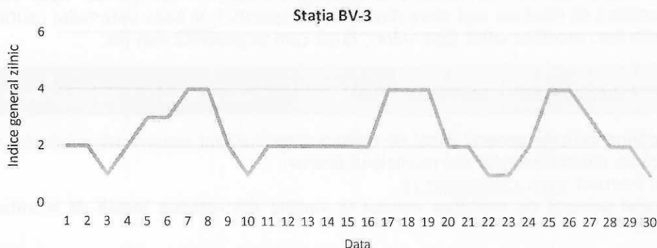
Figura 14. Evoluția indicelui general de calitate a aerului din stația BV-3
