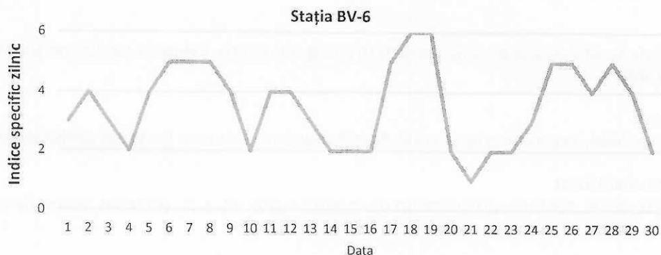
Figura 17. Evoluția indicelui general de calitate a aerului din stația BV-6
