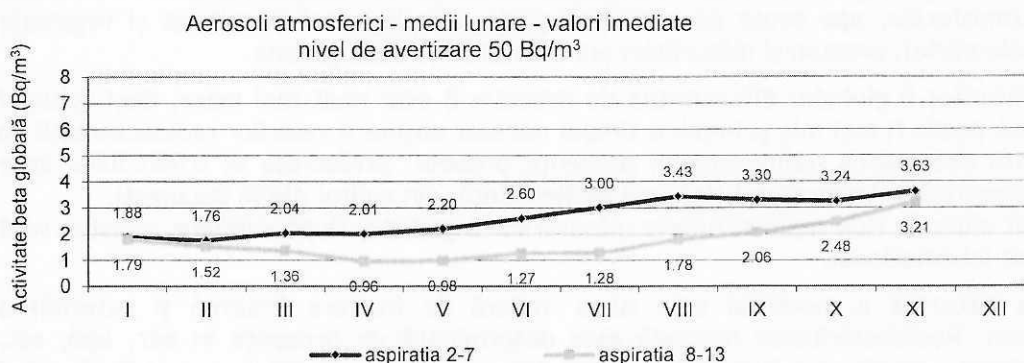
Figura 19. Activitatea beta globală pentru aerosoli atmosferici
