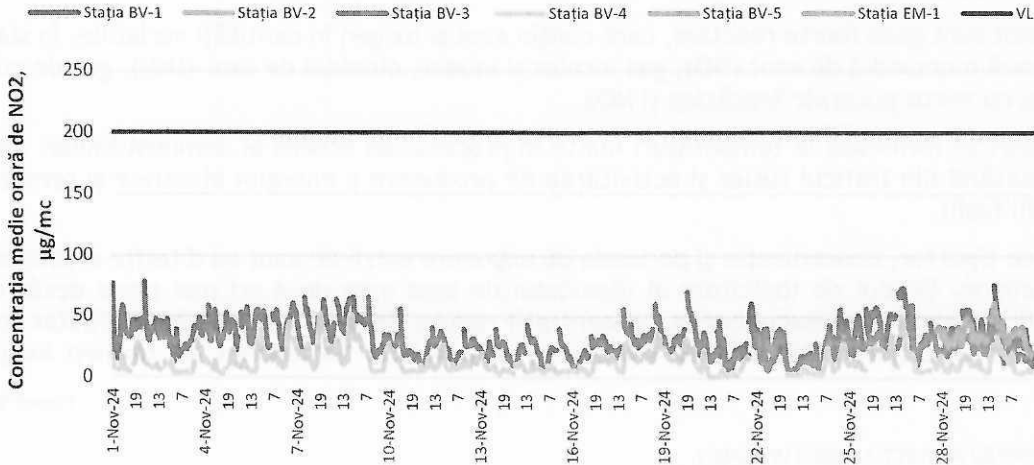
Figura 3. Concentrații medii orare de NO 2 în luna noiembrie 2024
