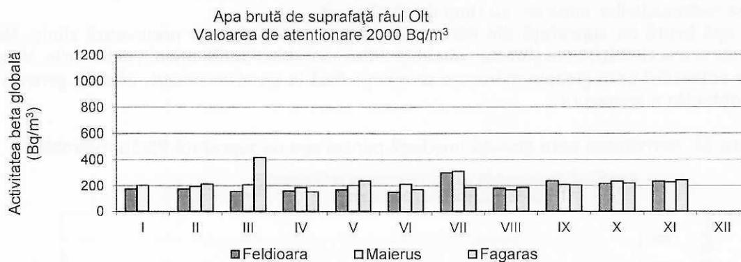
Fig. 25. Activitatea beta globală la 5 zile pentru apa de suprafață Râul Olt
