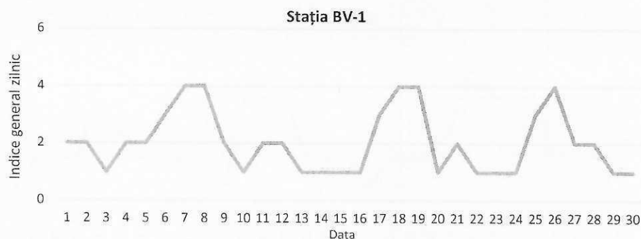
Figura 12. Evoluția indicelui general de calitatea aerului din stația BV-1
