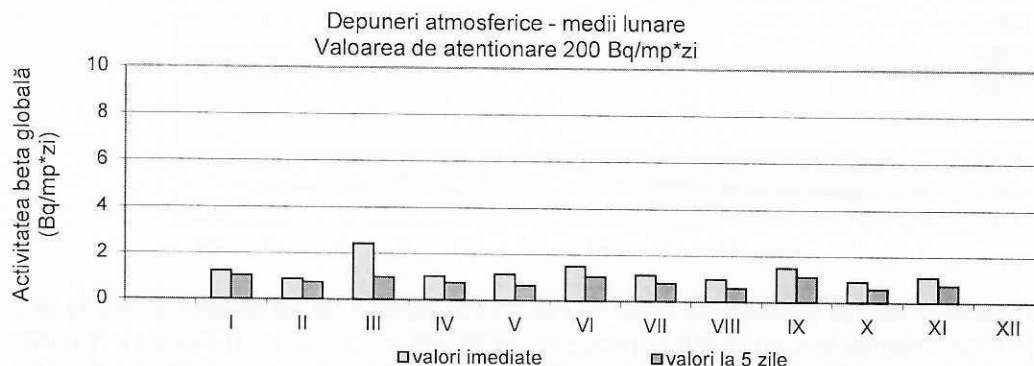
Figura 22. Activitatea beta globală pentru depuneri atmosferice
