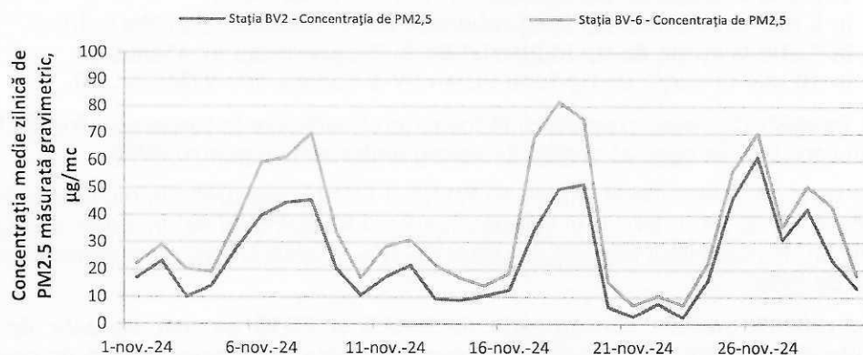
Figura 10. Evoluția concentrațiilor medii zilnice de PM 2,5 (gravimetric) în luna noiembrie 2024
