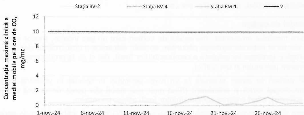
Figura 4. Concentrația maximă a mediei mobile pe 8 ore de CO în luna noiembrie 2024
