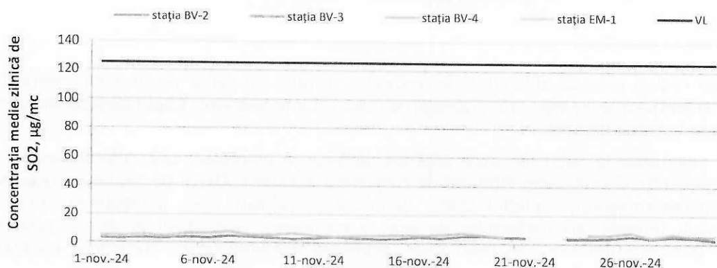
Figura 1. Evoluția mediilor zilnice de SO 2 în luna noiembrie 2024
