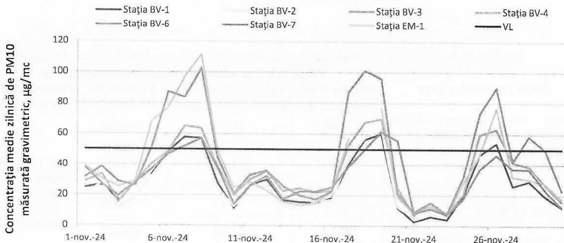
Figura 7. Evoluția concentrațiilor medii zilnice de PM 10 (gravimetric) în luna noiembrie 2024
