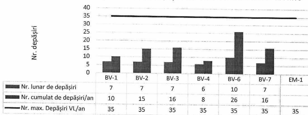
Figura 11. Numărul lunar și cumulat de depășiri ale valorii limită zilnice la PM10
