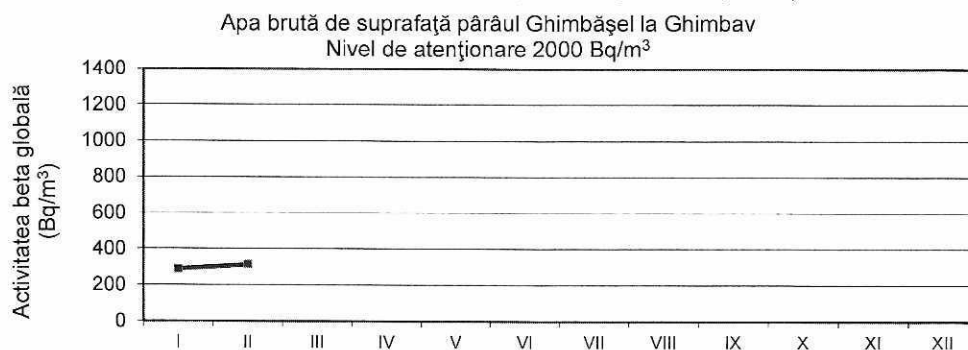
Figura 26. Activitatea beta globală imediată pentru apa de suprafață Pârâul Ghimbășel
