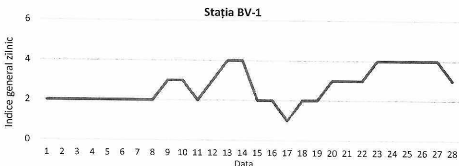
Figura 15. Evoluția indicelui general de calitate a aerului din stația BV-1
