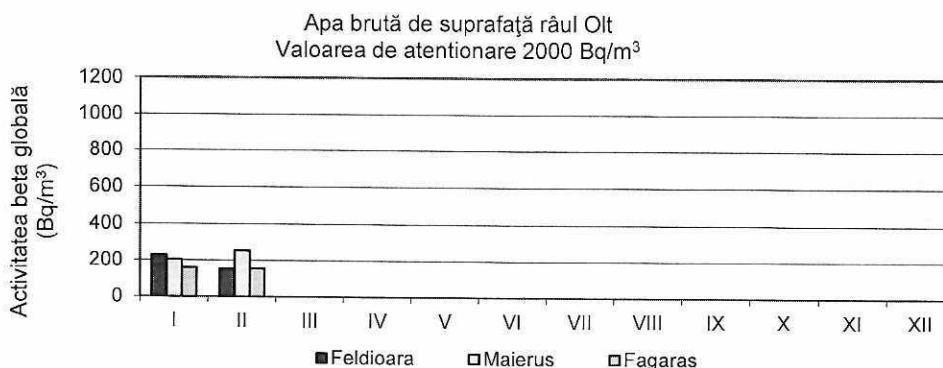
Fig. 28. Activitatea beta globală la 5 zile pentru apa de suprafață Râul Olt
