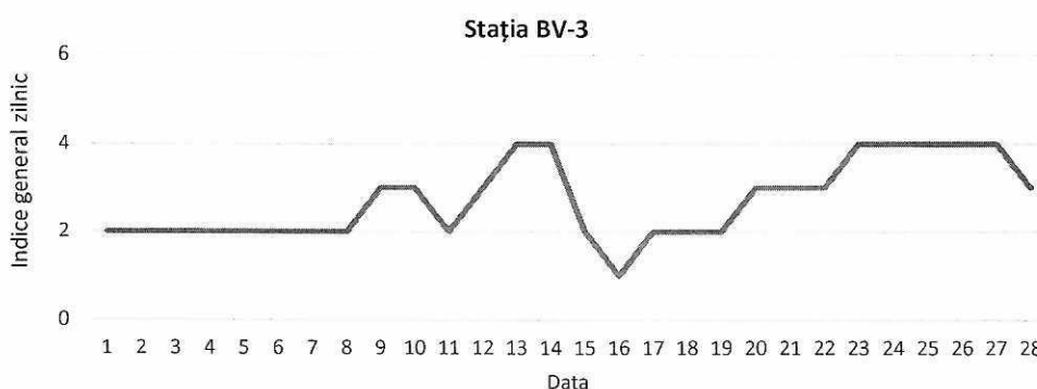
Figura 17. Evoluția indicelui general de calitate a aerului din stația BV-3
