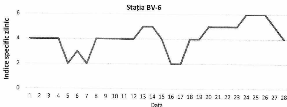
Figura 20. Evoluția indicelui general de calitate a aerului din stația BV-6
