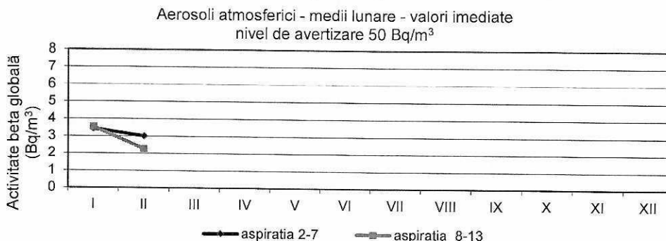
Figura 22. Activitatea beta globală pentru aerosoli atmosferici
