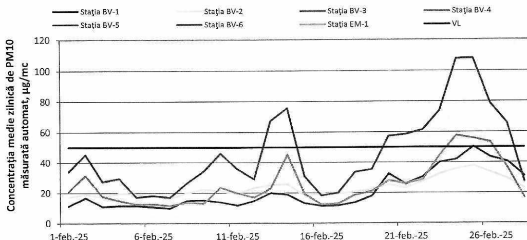
Figura 12. Evoluția concentrațiilor medii zilnice de PM 10 automat în luna februarie 2025
