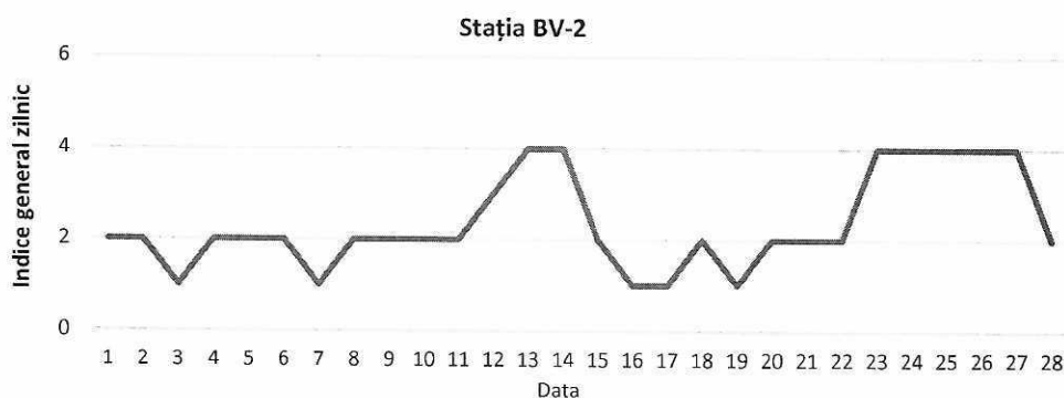
Figura 16. Evoluția indicelui general de calitate a aerului din stația BV-2
