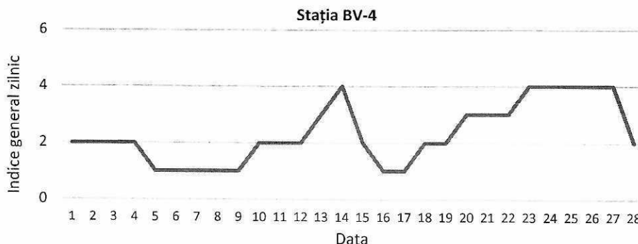
Figura 18. Evoluția indicelui general de calitate a aerului din stația BV-4
