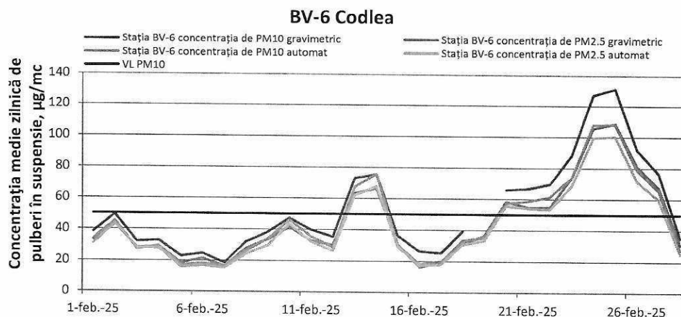
Figura 14. Evoluția concentrațiilor medii zilnice de PM10 gravimetric și automat și PM2,5 gravimetric și automat în stația de fond urban BV-6 în luna februarie 2025
