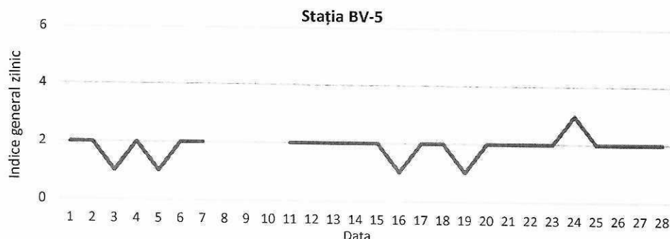
Figura 19. Evoluția indicelui general de calitate a aerului din stația BV-5
