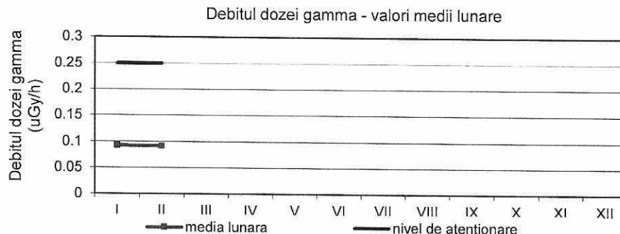
Figura 24. Debitul dozei gamma
