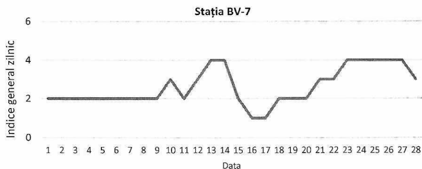
Figura 21. Evoluția indicelui general de calitate a aerului din stația BV-7
