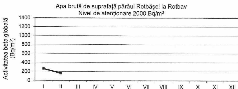
Figura 27. Activitatea beta globală la 5 zile pentru apa de suprafață-Pârâul Rotbășel
