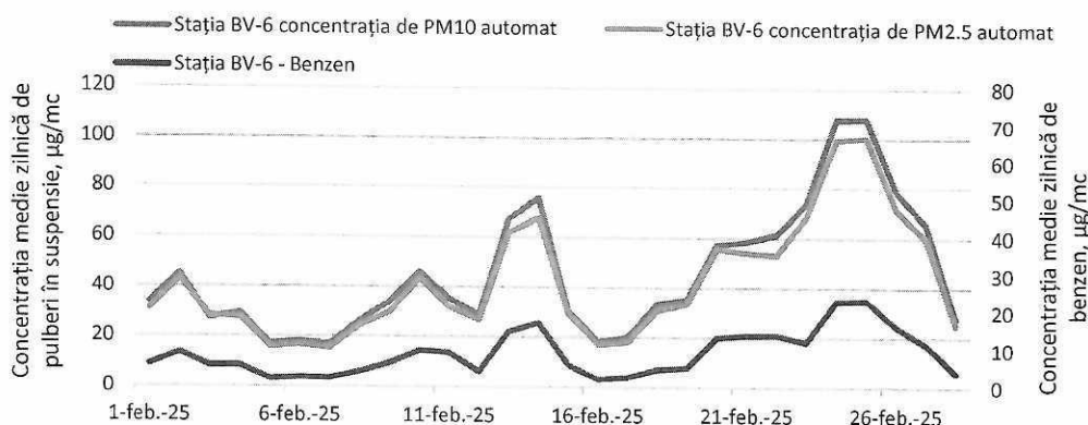
Figura 9. Evoluția concentrațiilor medii zilnice de benzen și pulberi în suspensie în luna februarie 2025
