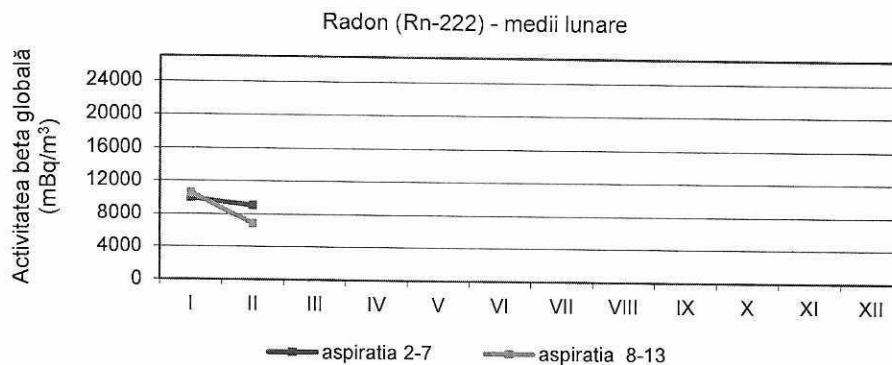
Figura 23. Activitatea calculată a Radonului
