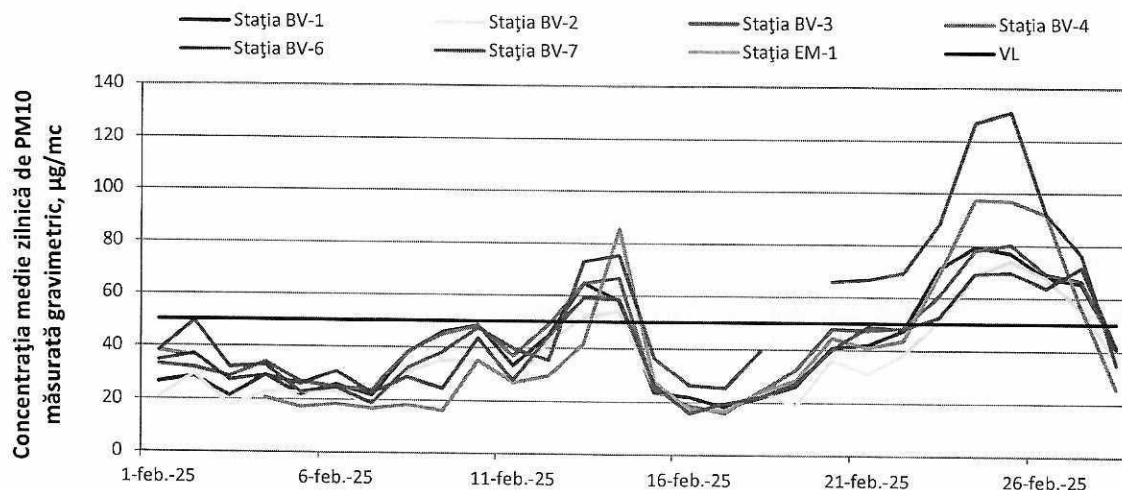
Figura 10. Evoluția concentrațiilor medii zilnice de PM 10 (gravimetric) în luna februarie 2025
