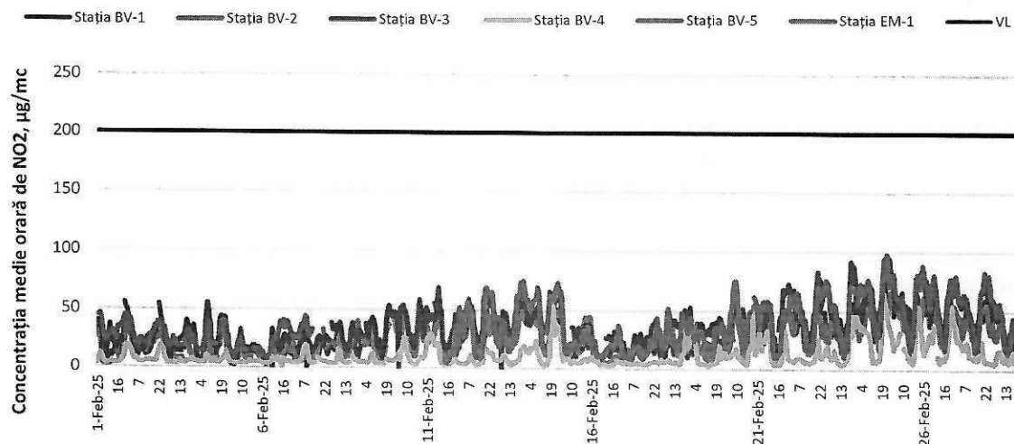
Figura 3. Concentrații medii orare de NO 2 în luna februarie 2025
