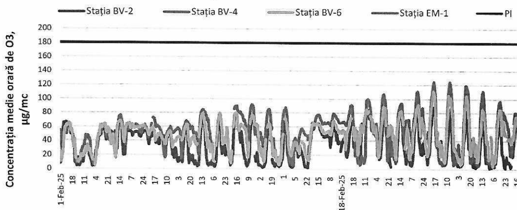
Figura 6. Evoluția concentrațiilor medii orare de O 3 în luna februarie 2025
