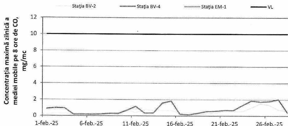
Figura 4. Concentrația maximă a mediei mobile pe 8 ore de CO în luna februarie 2025
