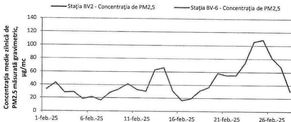
Figura 13. Evoluția concentrațiilor medii zilnice de PM 2,5 (gravimetric) în luna februarie 2025
