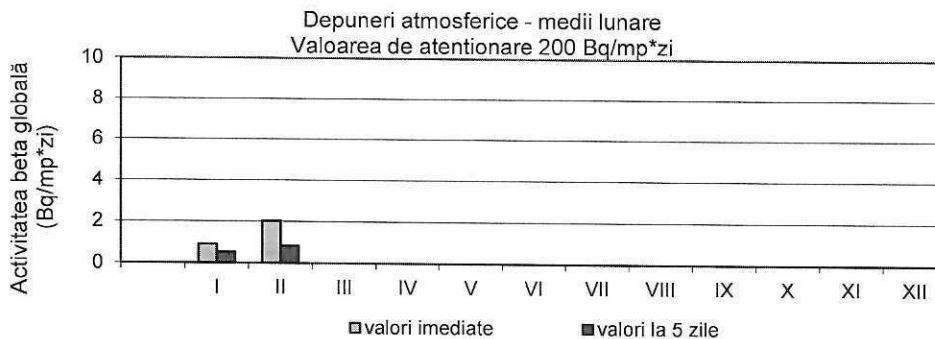
Figura 25. Activitatea beta globală pentru depuneri atmosferice
