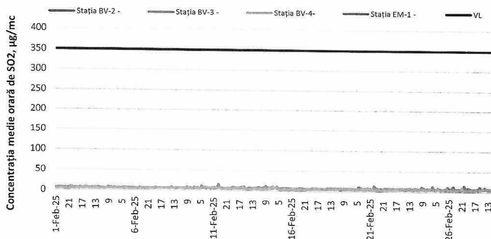
Figura 2. Evoluția mediilor orare de SO 2 în luna februarie 2025
