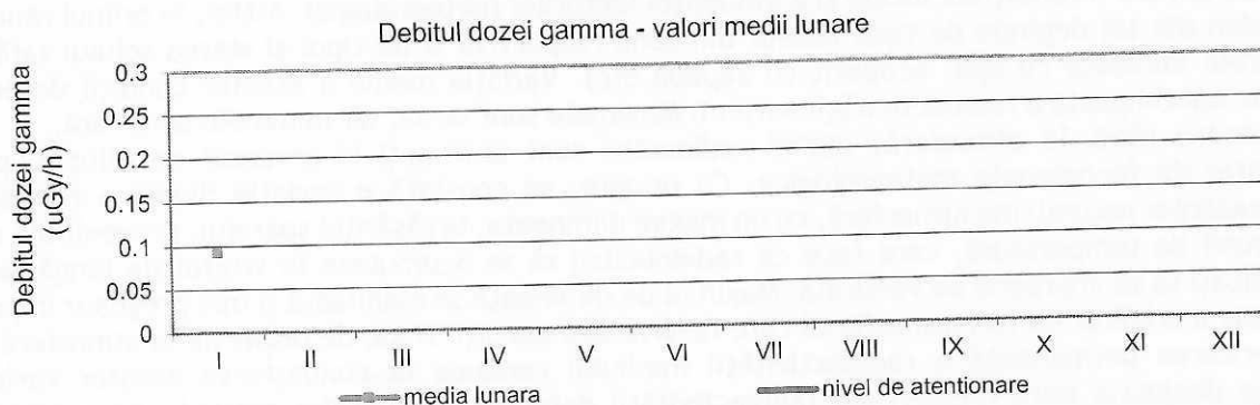
Figura 24. Debitul dozei gamma
