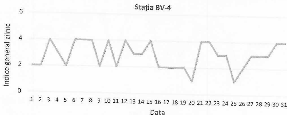
Figura 18. Evoluția indicelui general de calitate a aerului din stația BV-4
