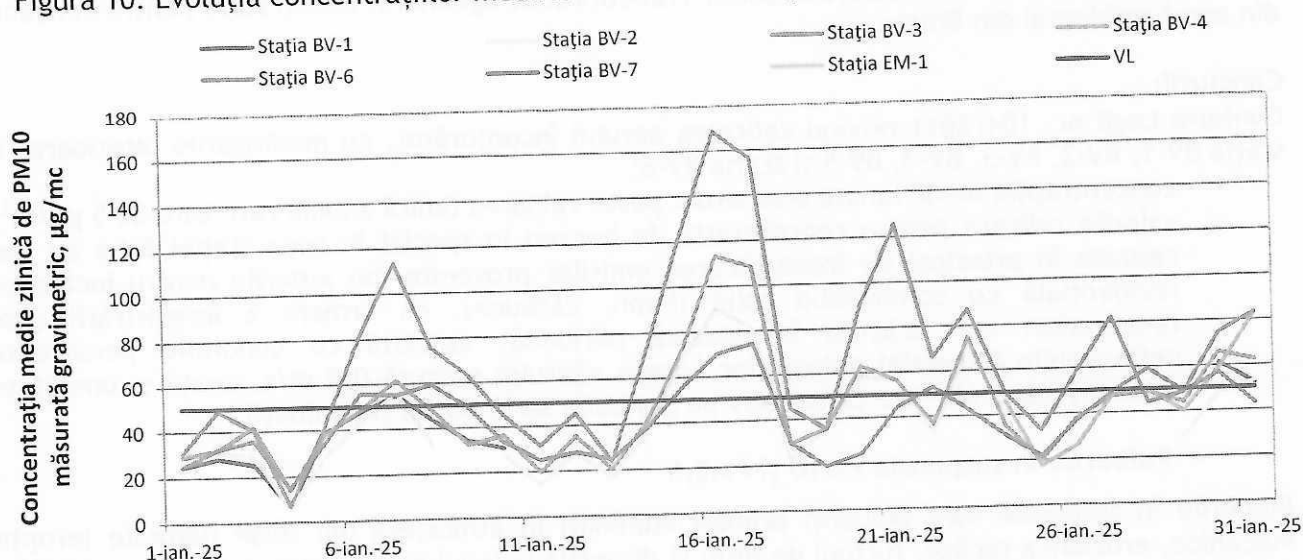
Figura 10. Evoluția concentrațiilor medii zilnice de PM 10 (gravimetric) în luna ianuarie 2025
