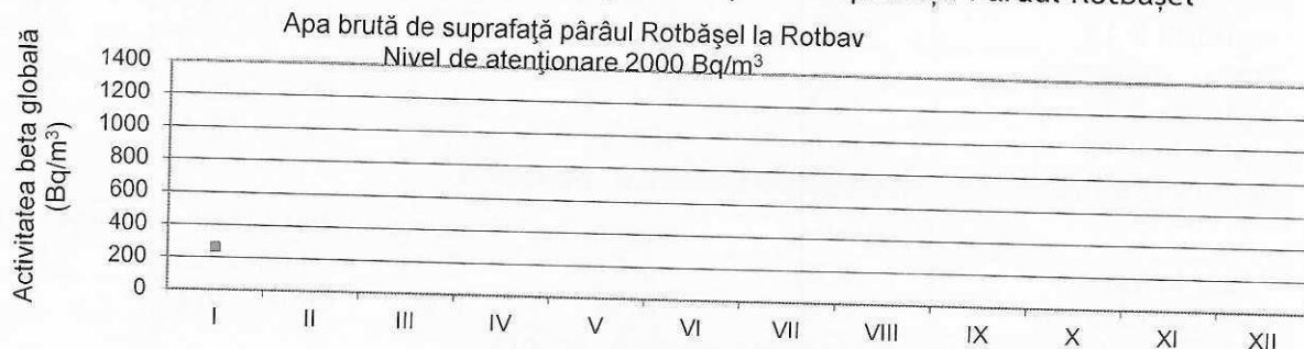
Figura 27. Activitatea beta globală la 5 zile pentru apa de suprafață-Pârâul Rotbășel
