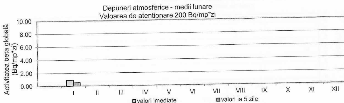
Figura 25. Activitatea beta globală pentru depuneri atmosferice
