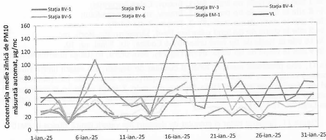
Figura 12. Evoluția concentrațiilor medii zilnice de PM 10 automat în luna ianuarie 2025
