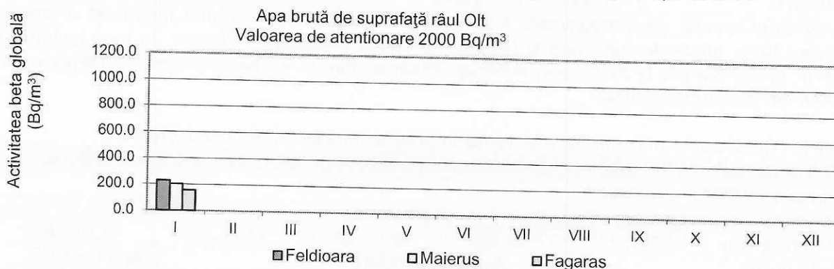
Fig. 28. Activitatea beta globală la 5 zile pentru apa de suprafață Râul Olt
