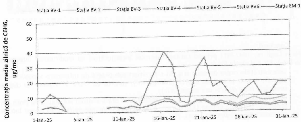
Figura 7. Evoluția concentrațiilor medii orare de benzen în luna ianuarie 2025
