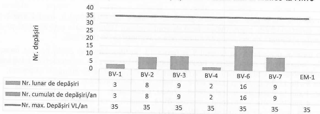
Figura 11. Numărul lunar și cumulat de depășiri ale valorii limită zilnice la PM10
