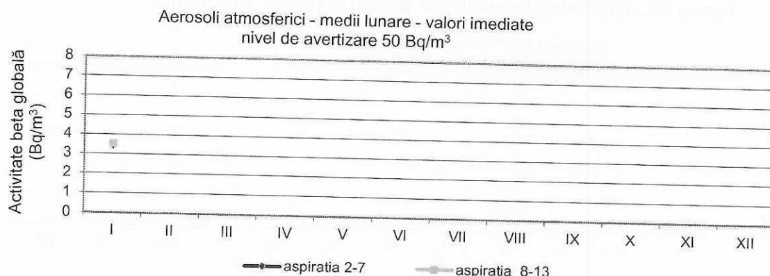
Figura 22. Activitatea beta globală pentru aerosoli atmosferici
