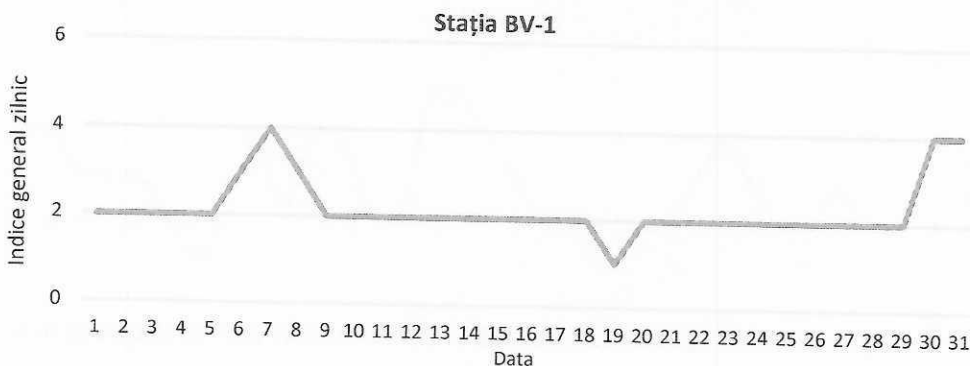
Figura 15. Evoluția indicelui general de calitate a aerului din stația BV-1
