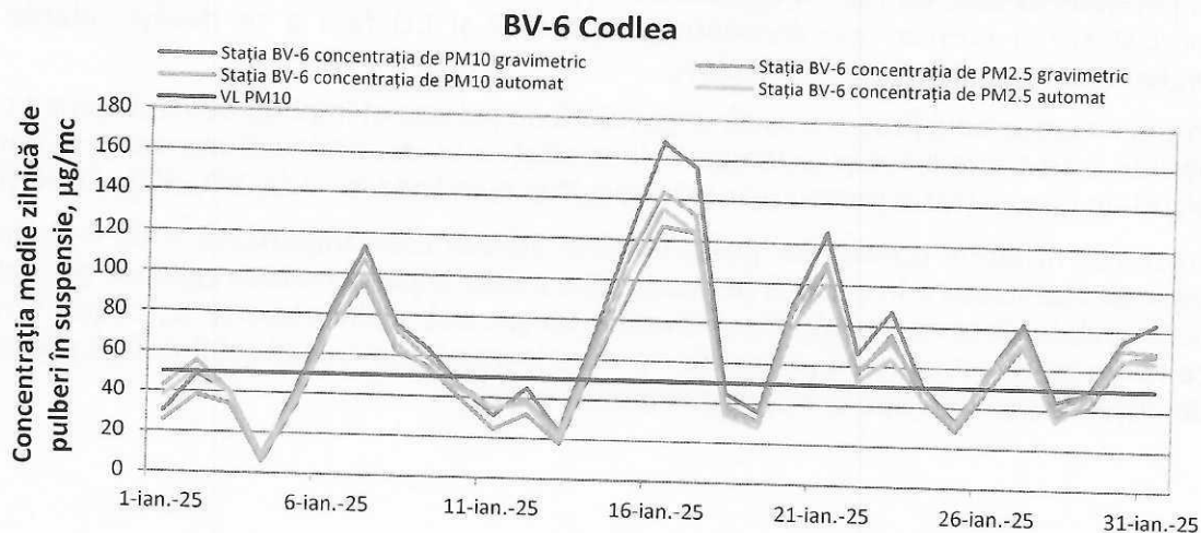
Figura 14. Evoluția concentrațiilor medii zilnice de PM10 gravimetric și automat și PM2,5 gravimetric și automat în stația de fond urban BV-6 în luna ianuarie 2025
