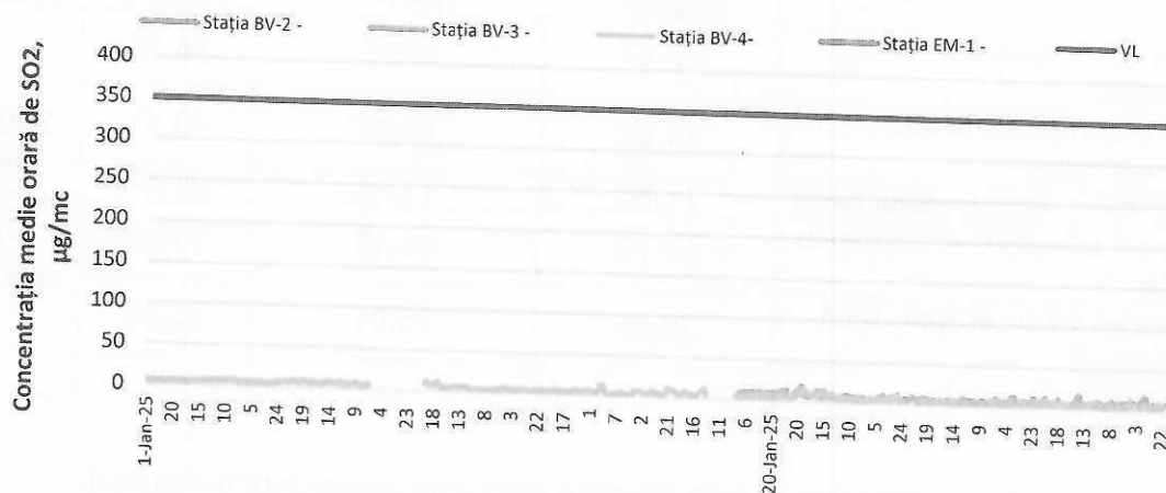
Figura 2. Evoluția mediilor orare de SO 2 în luna ianuarie 2025
