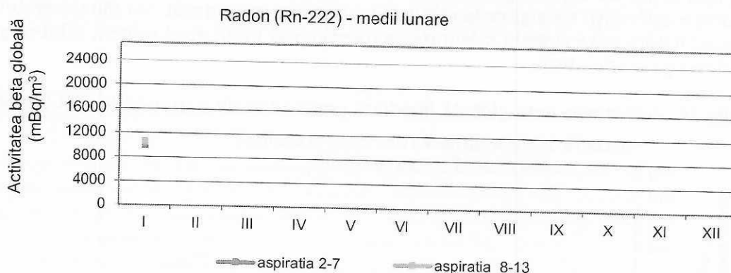
Figura 23. Activitatea calculată a Radonului
