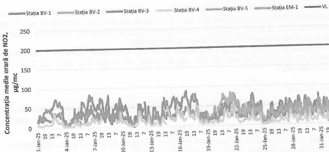
Figura 3. Concentrații medii orare de NO 2 în luna ianuarie 2025
