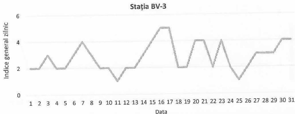
Figura 17. Evoluția indicelui general de calitate a aerului din stația BV-3
