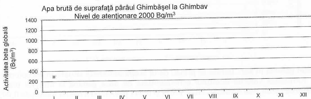
Figura 26. Activitatea beta globală imediată pentru apa de suprafață Pârâul Ghimbășel
