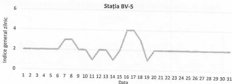
Figura 19. Evoluția indicelui general de calitate a aerului din stația BV-5
