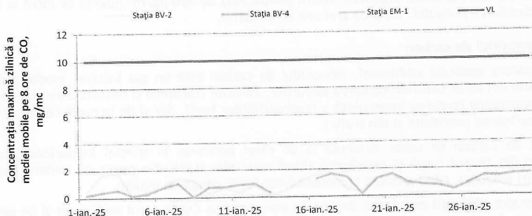
Figura 4. Concentrația maximă a mediei mobile pe 8 ore de CO în luna ianuarie 2025
