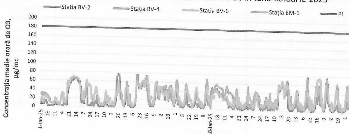
Figura 6. Evoluția concentrațiilor medii orare de O_3 în luna ianuarie 2025
