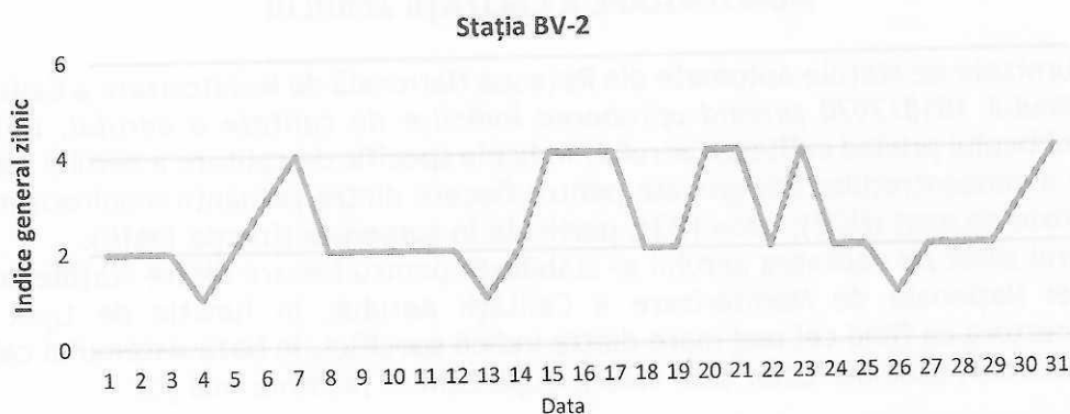
Figura 16. Evoluția indicelui general de calitate a aerului din stația BV-2
